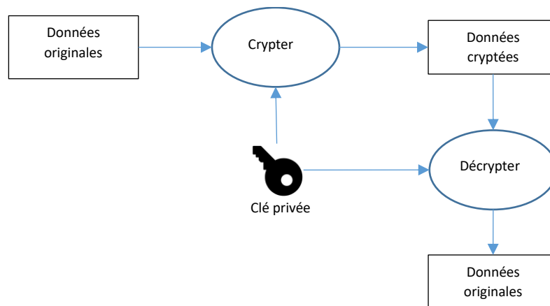
Figure 1: Chiffrement symétrique
