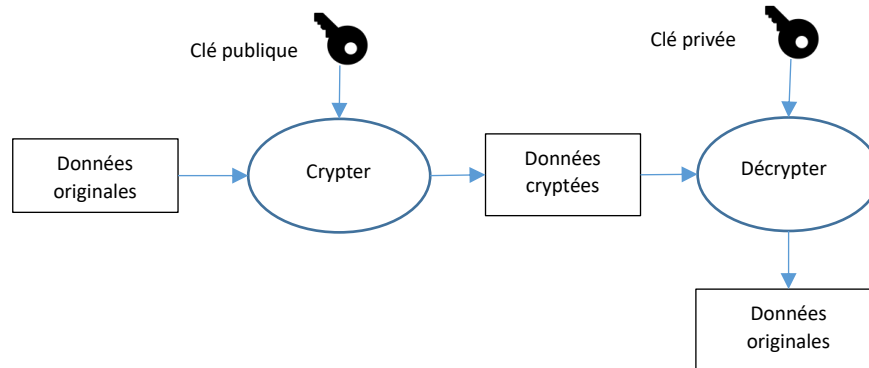
Figure 2: Chiffrement asymétrique
